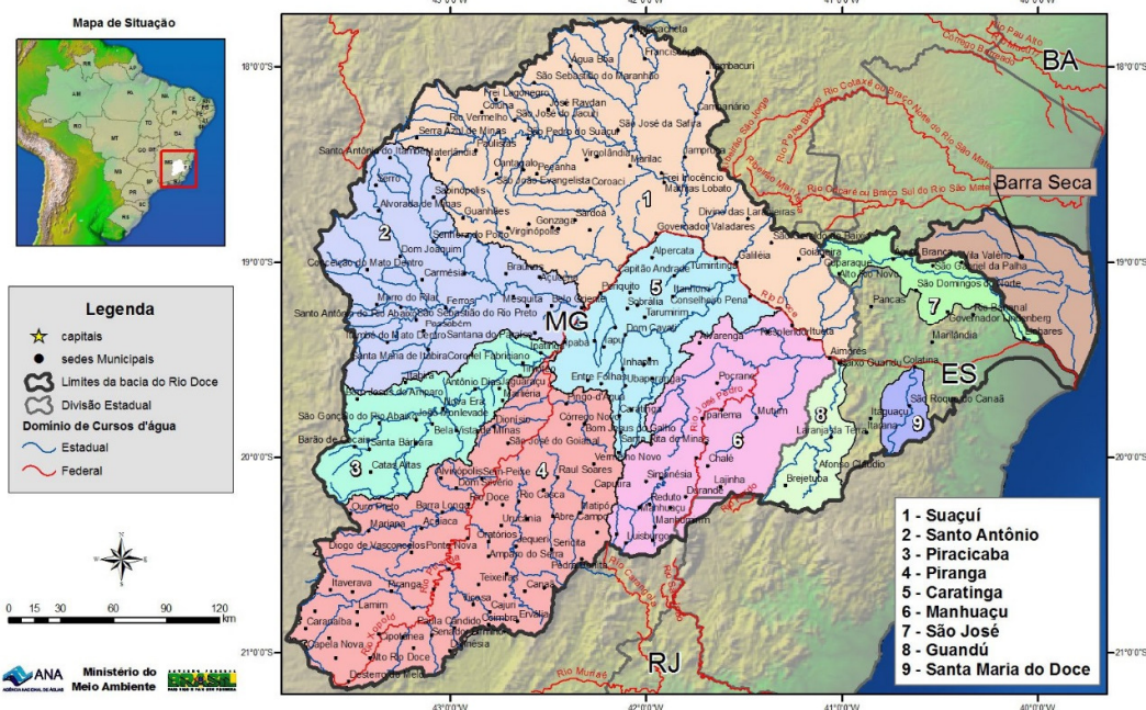
FIGURA 1. Mapa da Bacia Hidrográfica do Rio Doce, com suas sub-bacias.
