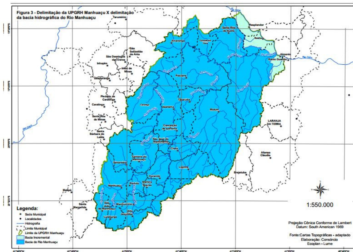
FIGURA 3. Bacia da UPRH Manhuaçu, destacando a bacia do Rio Manhuaçu (azul) e a Bacia incremental (verde) (Fonte: Plano Diretor da Bacia do Rio Doce)
